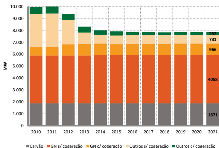
Fig. 54 Potência instalada - não renovável
