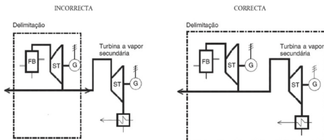
Figura 4 — Delimitação do sistema quando existem turbinas a vapor secundárias (ST: Turbina a Vapor), figura extraída da Decisão da Comissão 2008/952/CE de 19 de novembro de 2008 que estabelece orientações circunstanciadas para implementação e aplicação do Anexo II da Diretiva 2004/8/CE do Parlamento Europeu e do Conselho, de 11 de fevereiro de 2004.
