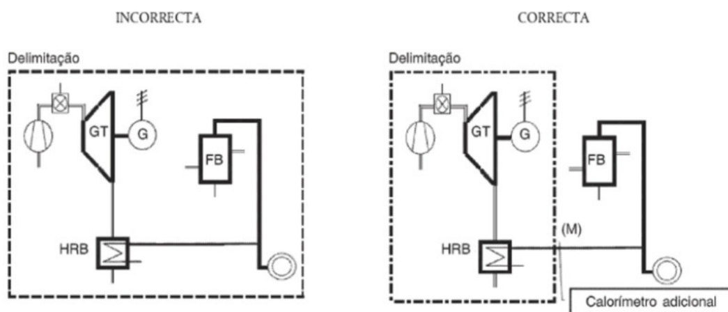
Figura 3 — Delimitação quando existem caldeiras auxiliares ou de reserva (GT: Turbina a gás, G: Gerador, FB: Caldeira a combustível, HRB: Caldeira de recuperação de calor); figura extraída da Decisão da Comissão 2008/952/CE de 19 de novembro de 2008 que estabelece orientações circunstanciadas para implementação e aplicação do Anexo II da Diretiva 2004/8/CE do Parlamento Europeu e do Conselho, de 11 de fevereiro de 2004.
